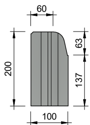
Linkeraanzicht
