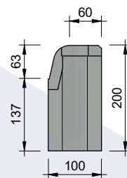
Rechteraanzicht
