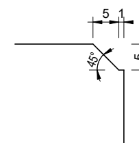
Vellingkant lange achterzijde 1 : 1
