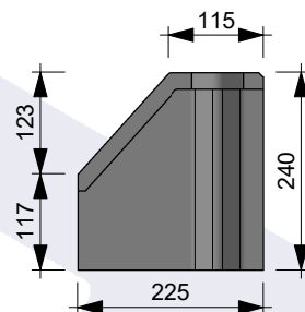
Rechteraanzicht
