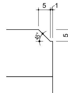
Vellingkant lange achterzijde 1:1
