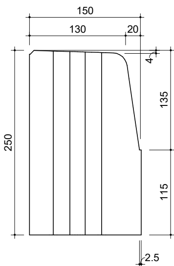
Linkeraanzicht met detail 1:5
