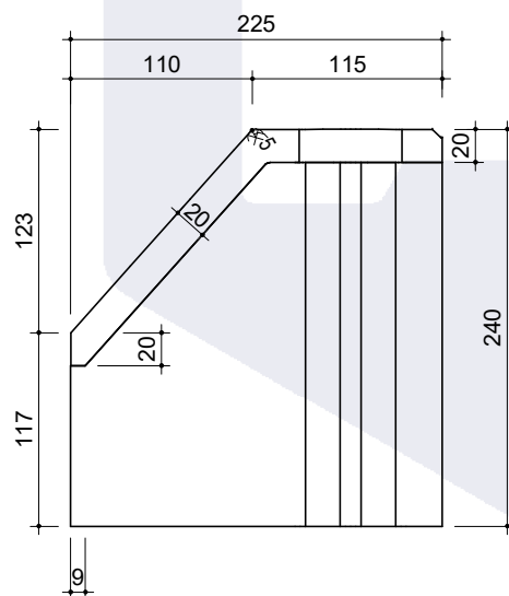
Rechteraanzicht met detail 1:5
