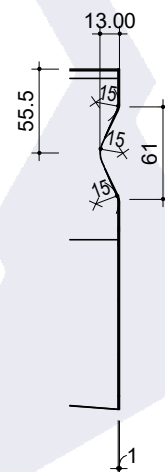
Detail verbinding rechts 1:5
