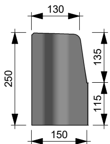
Linkeraanzicht
