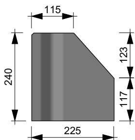
Linkeraanzicht
